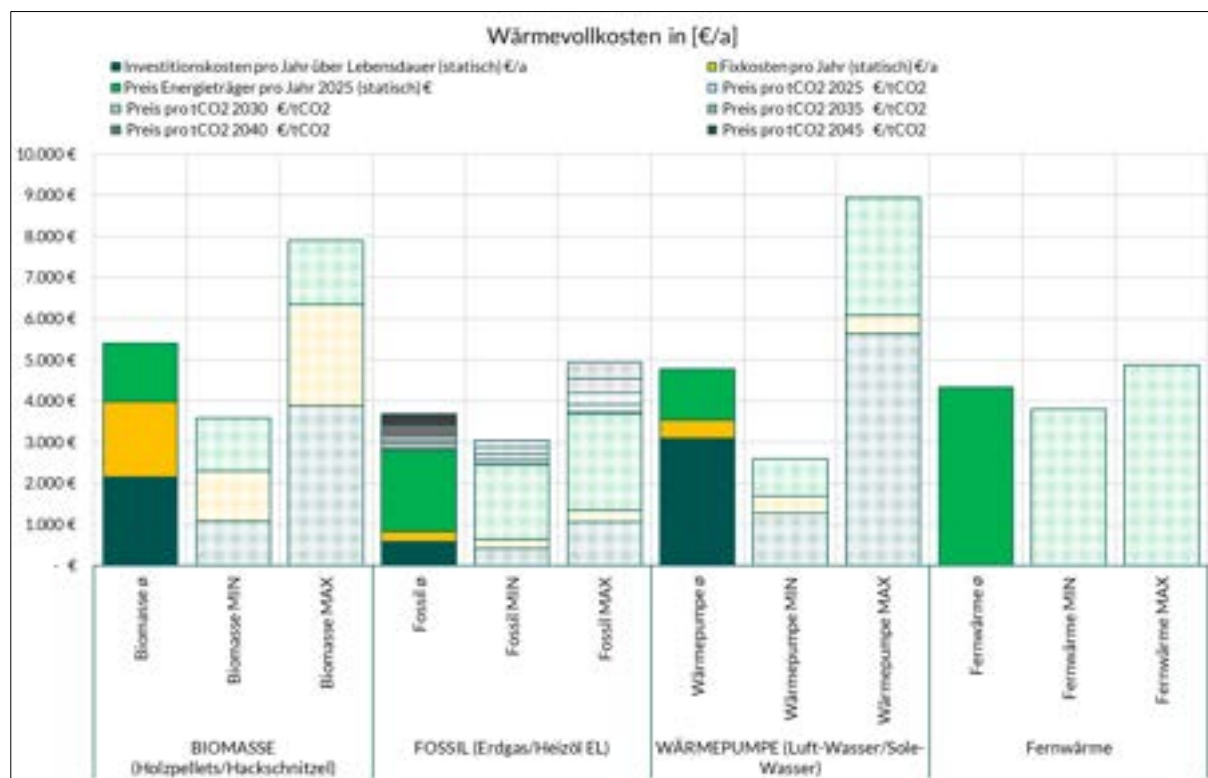
Abbildung 109: Wärmevollkosten - Verteilung Kostenarten (EFH - mittlerer Wärmebedarf)
