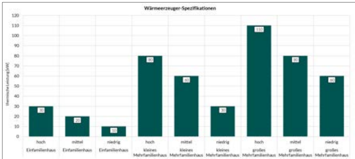
Abbildung 108: Wärmevollkosten – Wärmeerzeugerspezifikationen (Nennleistung)
