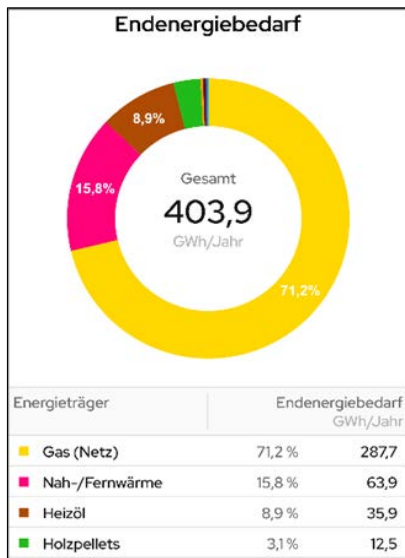
Abbildung 6: Endenergiebedarf Güstrow
